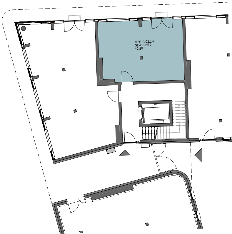
ERDGESCHOSS
